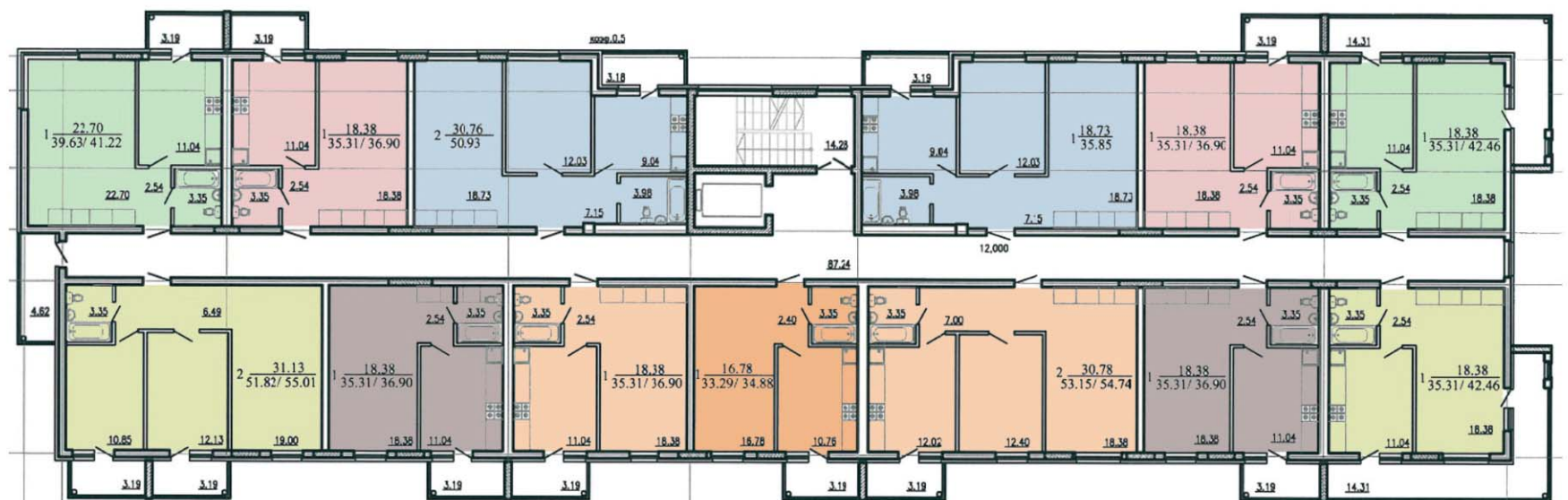
План типовой секции
