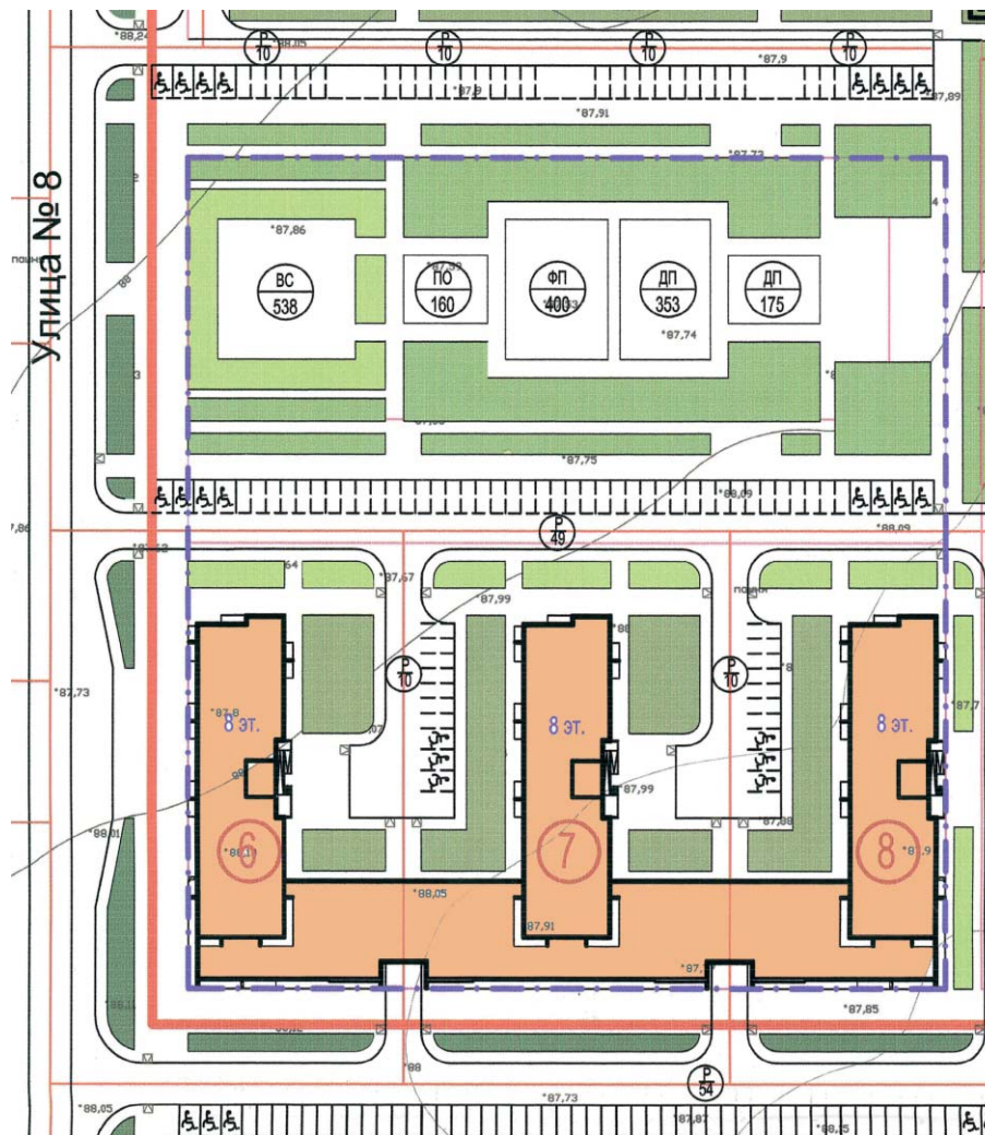
Схема генерального плана
